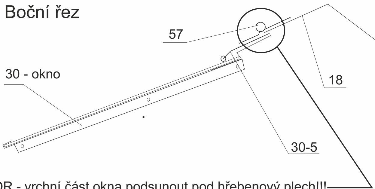
Konstrukce okna je podvlečena pod hřebenový plech (u přístaveb D a E horní střešní plech poz.32.)
