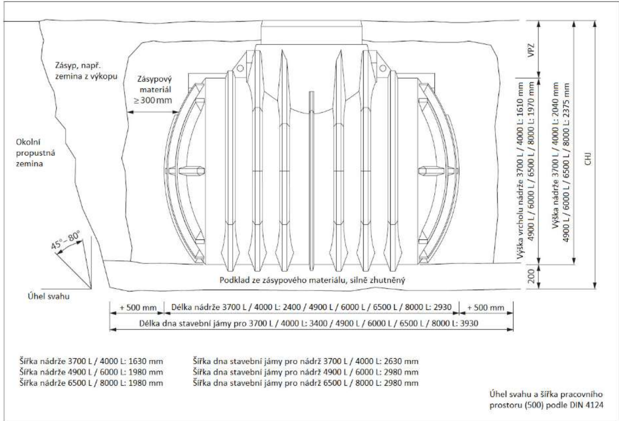
Obr. 2: Montážní velikosti
